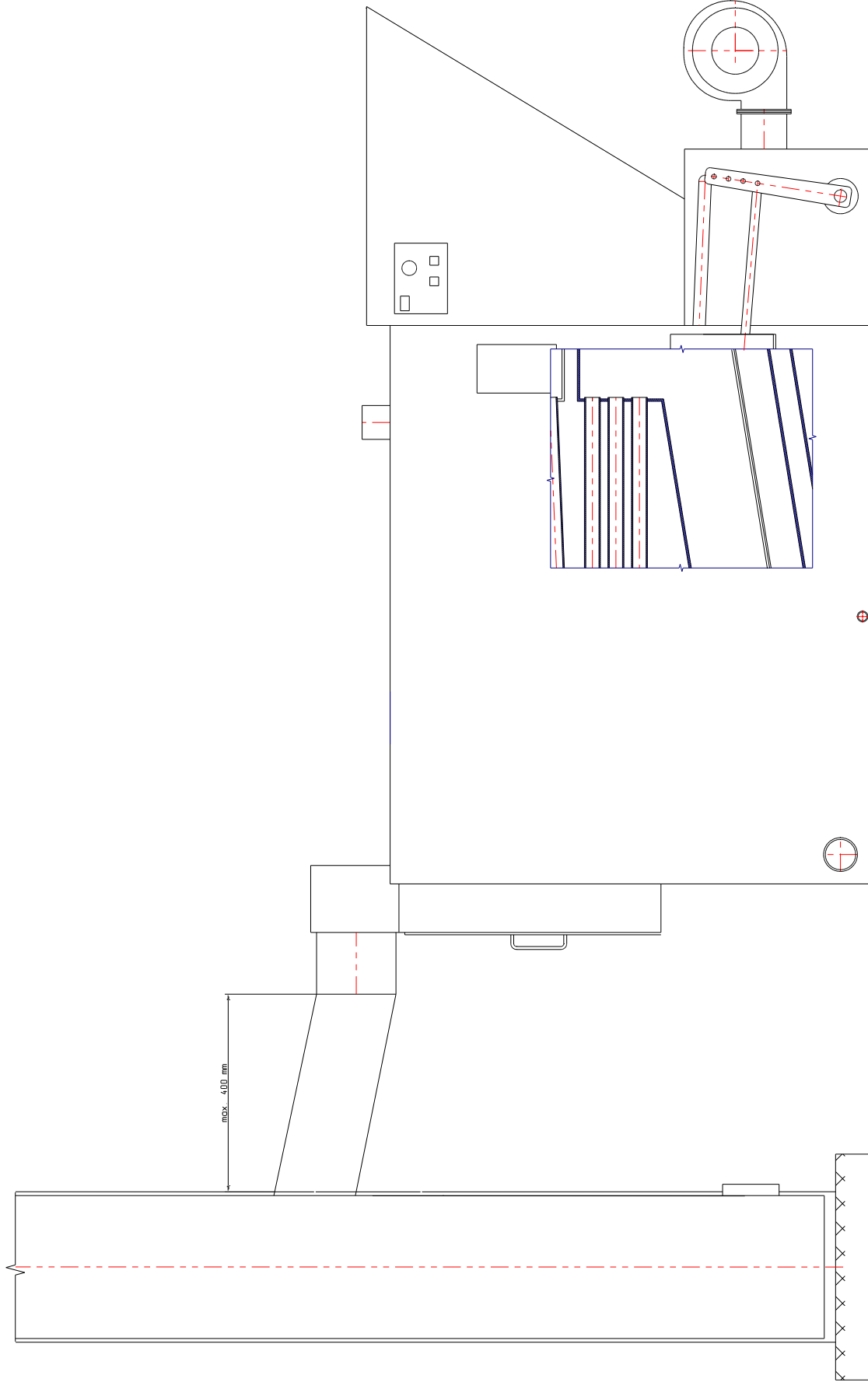
Rys.2 Schemat typowego podłączenia kotła KMK do przewodu kominowego.
